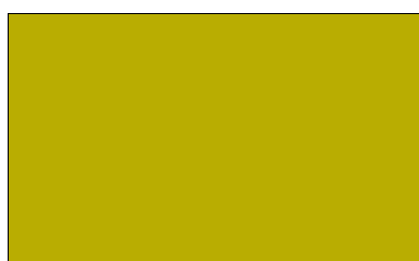
U15110 iguana
